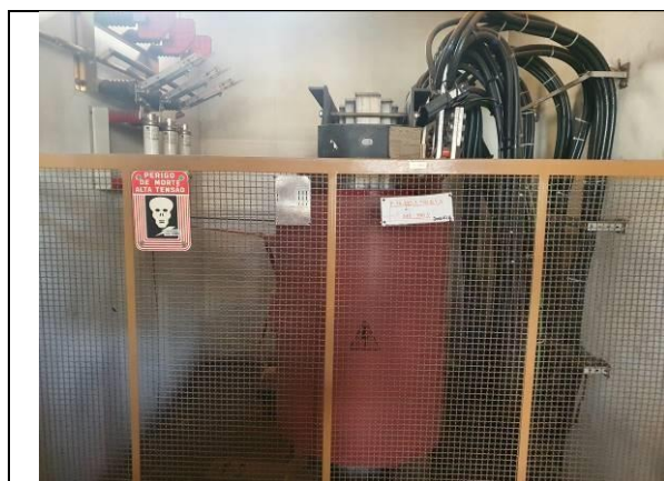
Item 1: Transformador trifásico, 3000 Kva, 13.000v. marca Mag.
